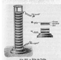
Fig. 315. — Pile de Volta.
